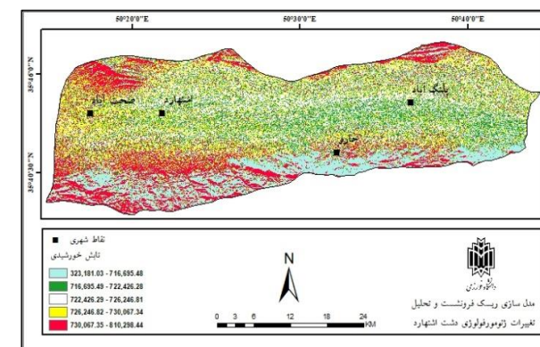
شکل ۱۴. نقشه تابش خورشیدی
