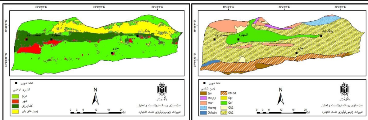
شکل ۱۰. نقشه کاربری اراضی
