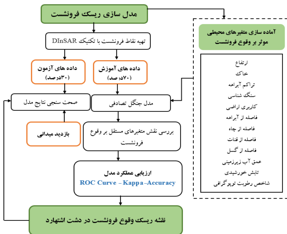
شکل ۲. نمودار روش کار مدل سازی ریسک خطر وقوع فرونشست با روش جنگل تصادفی
